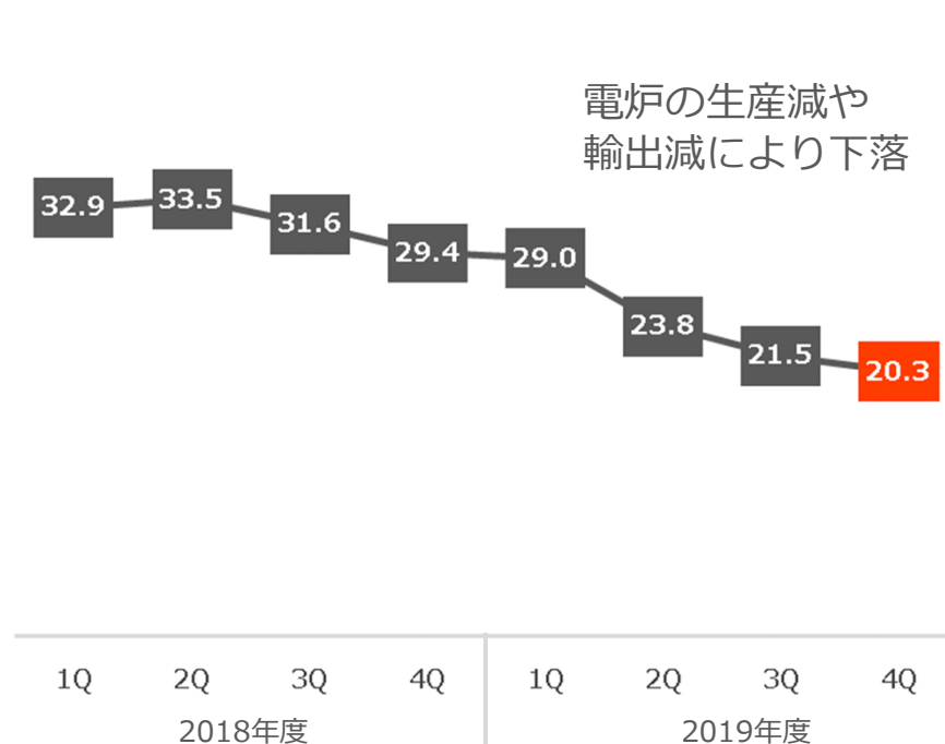
鉄スクラップ価格（円/kg） （H2炉前価格）
