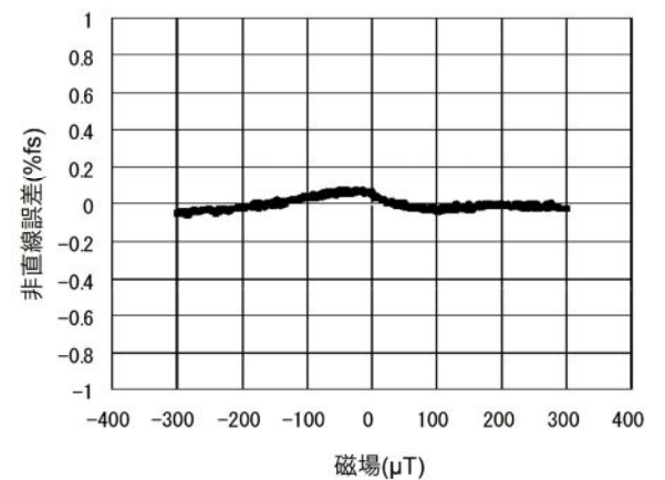
図2 直線性
