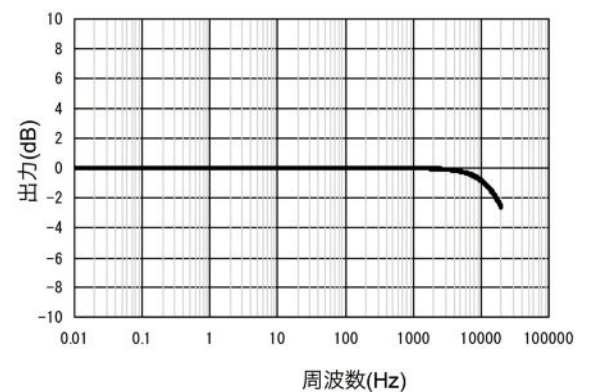
図3 周波数特性
